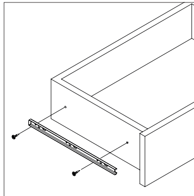
Ensamble de correderas con cajones.
