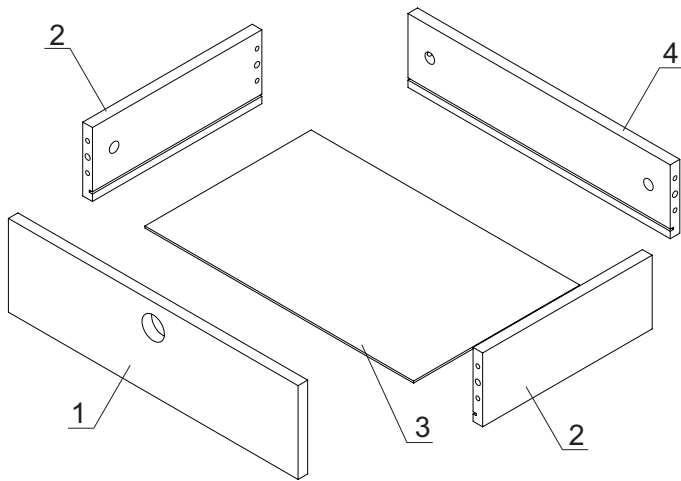
Ensamble fondo con laterales Minifix corto con caja y tarugo de 8 largo.
