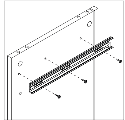
Ensamble de correderas con laterales.
