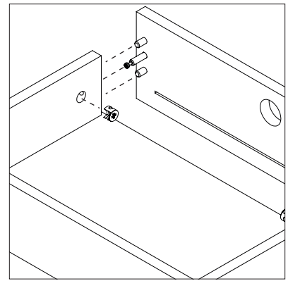
Ensamble tapa con laterales Minifix corto con caja y tarugo de 8 largo.
