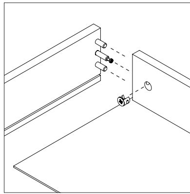
Ensamble fondo con laterales Minifix corto con caja y tarugo de 8 largo.
