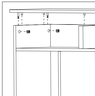
Ensamble tapa superior con laterales
