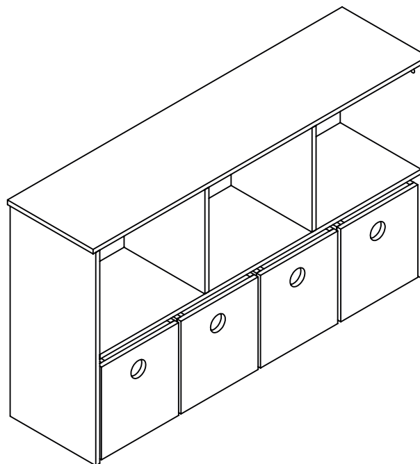
Ensamble tapa superior con laterales Minifix corto con caja y tarugo de 8 largo.
